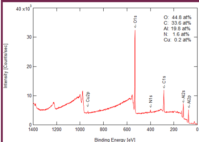
Fig-1 : Al表面の酸化膜のSurveyスペクトル
