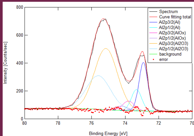
Fig-2 : Al表面の酸化膜の波形分離解析
